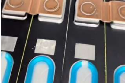
连接片焊接
