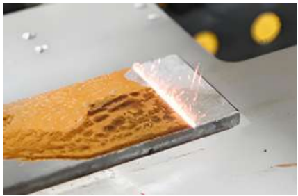
激光除污
